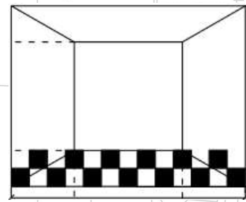
Det. 1 Esimerkki tyynyhidasteesta
