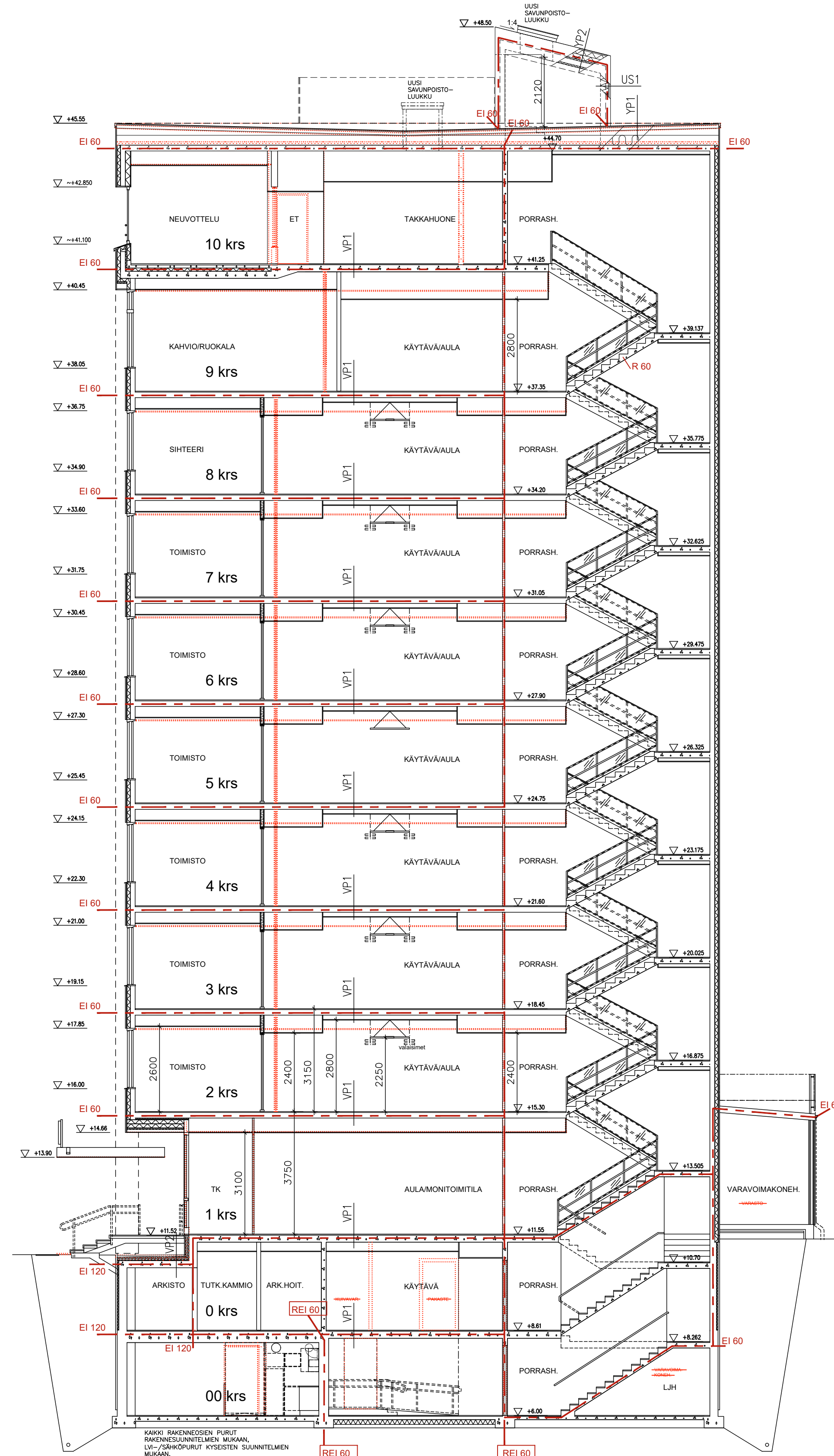
LEIKKAUS B-B KORKEUDET NN
