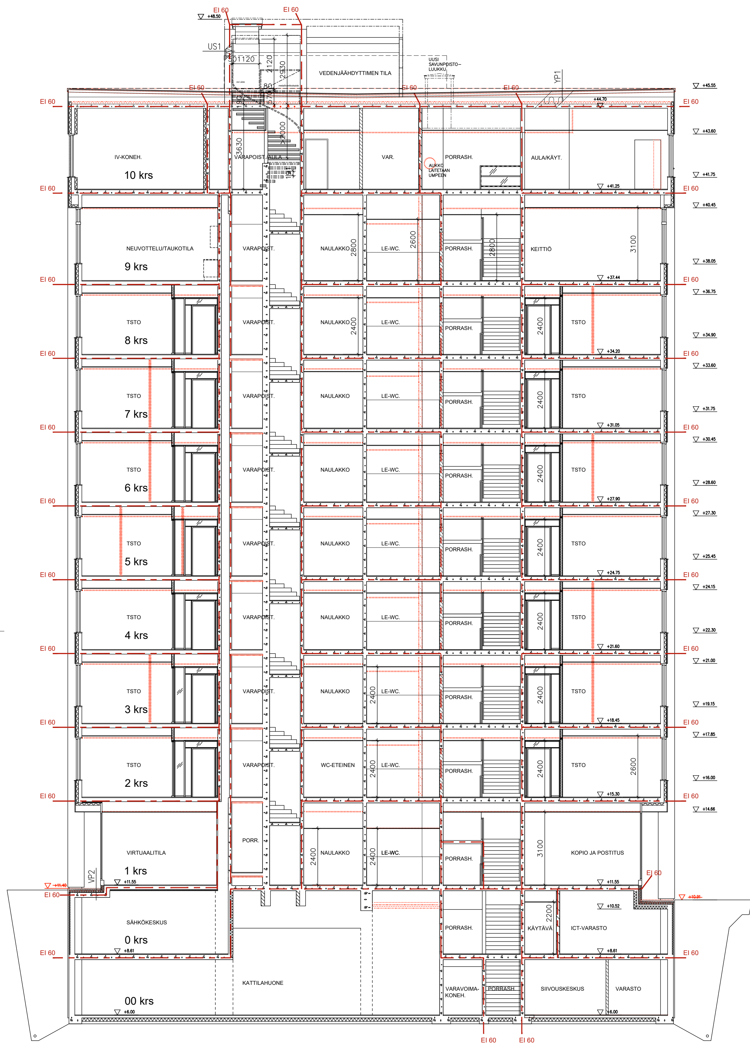
LEIKKAUS A-A KORKEUDET NN
